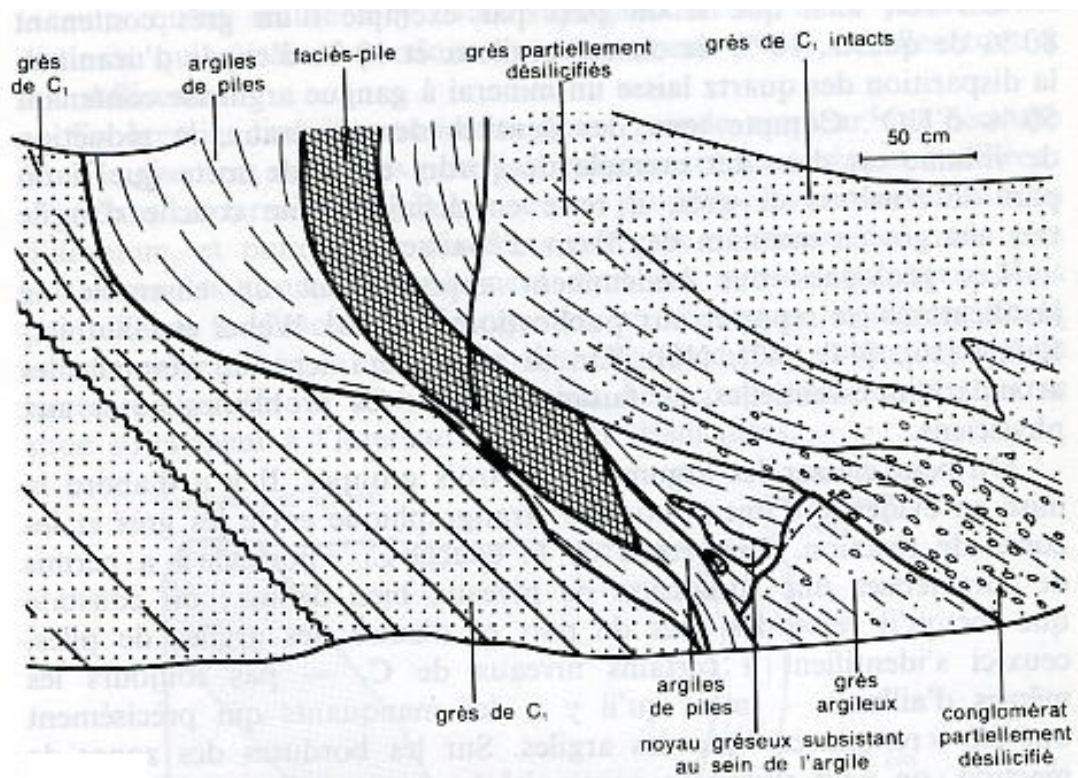
— Front du 30/9/76 (zones 5-6) (d'après [16]). On observe toute une série de transitions entre le réacteur et le minerai gréseux.
