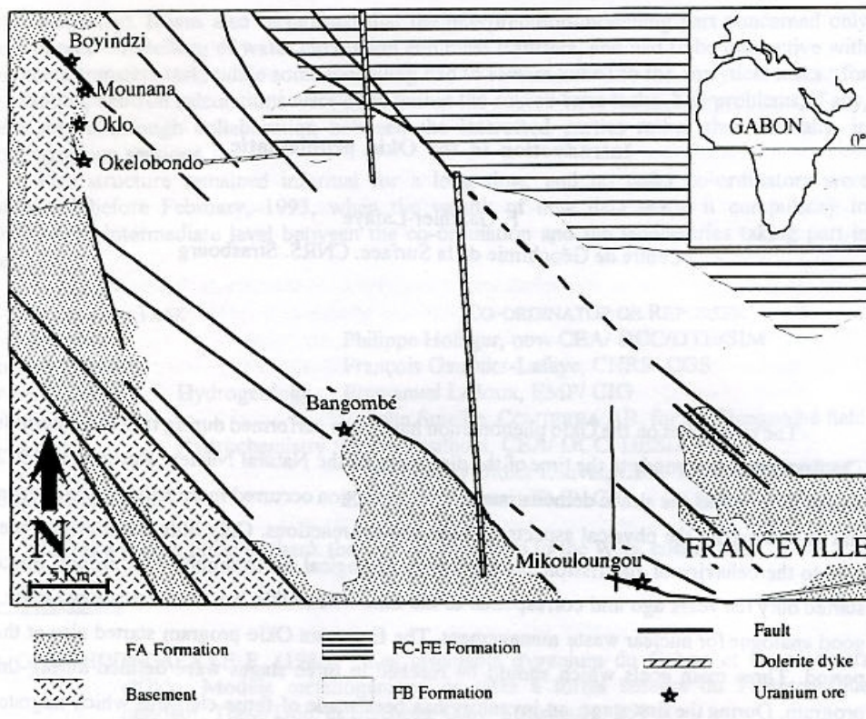
Figure 2 : Carte géologique du bassin de Franceville avec les gisements d'uranium
